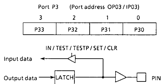
Figure1-2. Port P3
