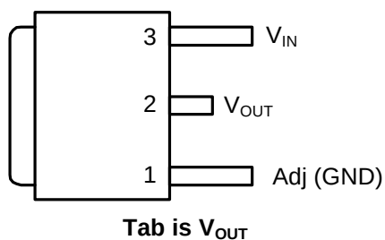
(3) TO220-3L
