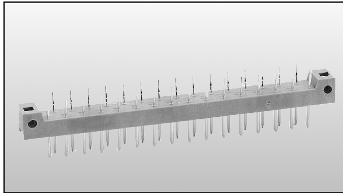
Stiftleiste mit geraden Einlötfüßen Sonderisoliertkörper Anschlußraster 3,8 mm
