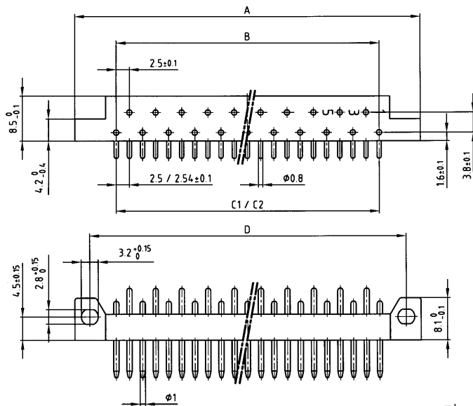
Leiterplattenbohrbild PCB-hole pattern
