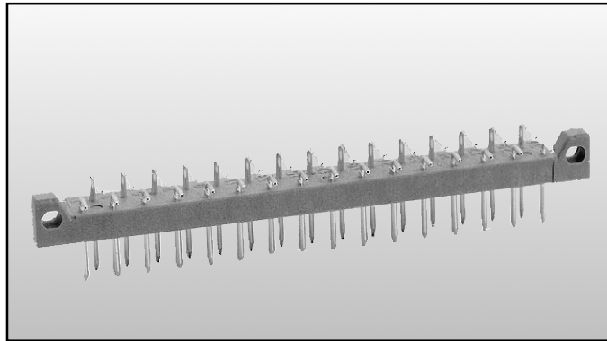
Stiftleiste mit abgewinkelten Einlötfitten Anschlußraster 2,5 und 2,54 mm
