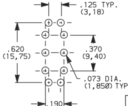
7201J1_BE2 DPDT
