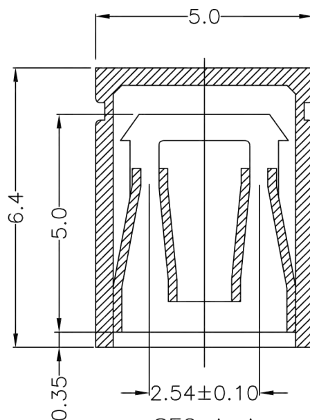
SEC A-A
