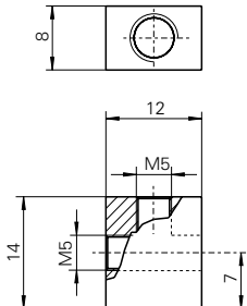
T-Stück (PT-300-M5)
