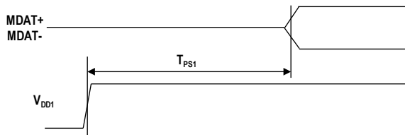
Figure 7. Data delay upon VDD1 startup
