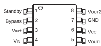
TS419IQT, TS419-xIQT: DFN8
