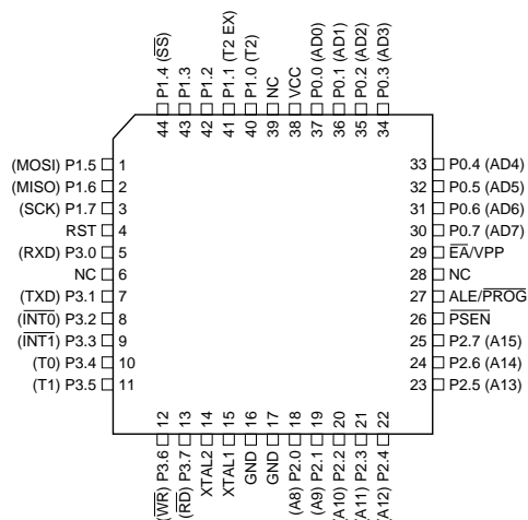
PQFP/TQFP
