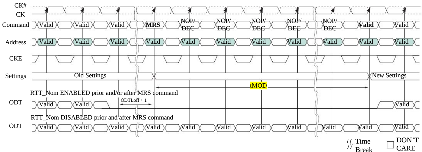
Figure 2.3.1b tMOD Timing
