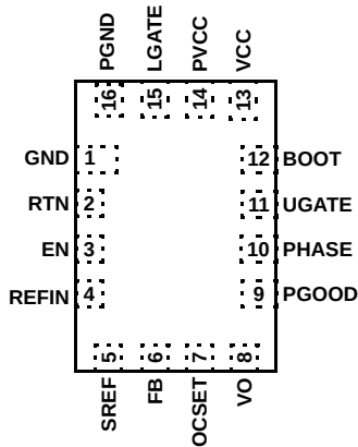
ISL95873 (16 LD 2.6X1.8 UTQFN) TOP VIEW
