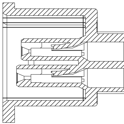
SECT A-A
