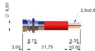
SOLDER LUG/FASTONS
