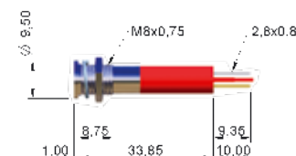
SOLDER LUG/FASTONS
