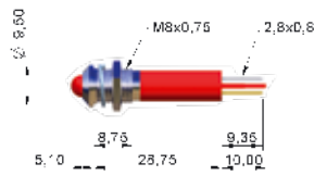
SOLDER LUG/FASTONS
