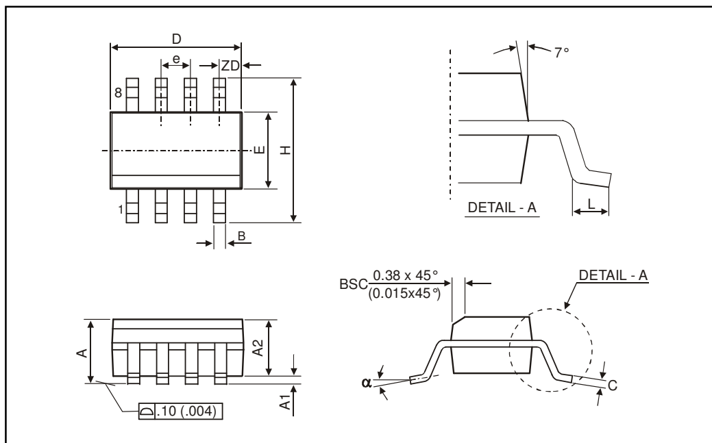
Fig. 19: SOIC8
