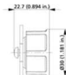
Katalog- Maßzeichnung
