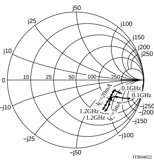
S22e : V_{CE}=-10V f=100MHz, 200 \text{ to } 1200MHz(200MHz \text{ step})
