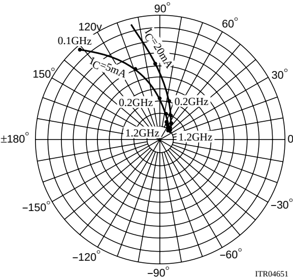
S21e : V_{CE}=-10V f=100MHz, 200 \text{ to } 1200MHz(200MHz \text{ step})
