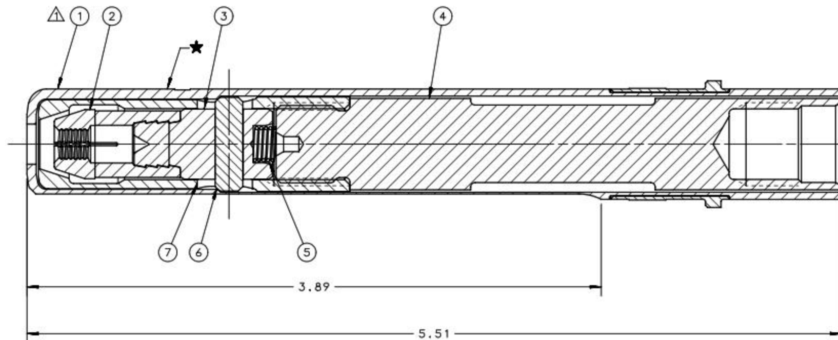
SECTION A-A
