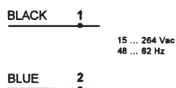
S5-1-G8
