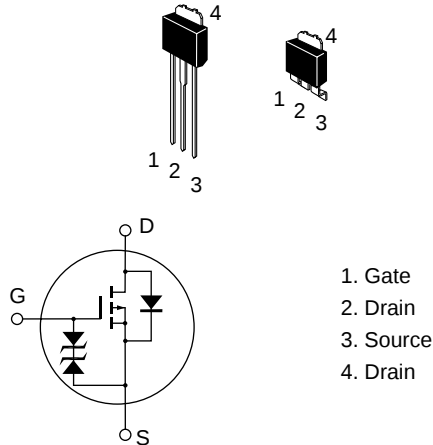
DPAK-2
