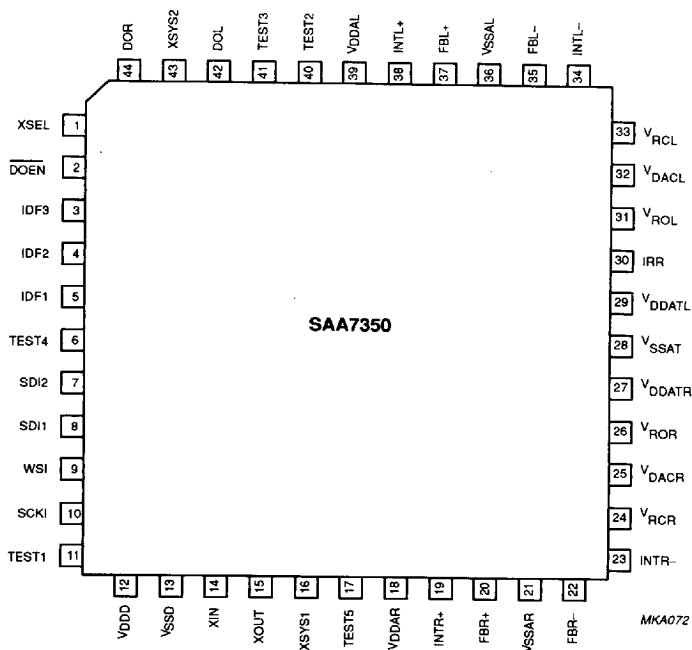
Fig.2 Pinning diagram.
