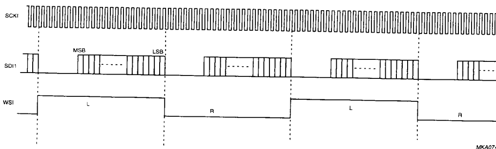
Fig.4 Sony serial input format.
