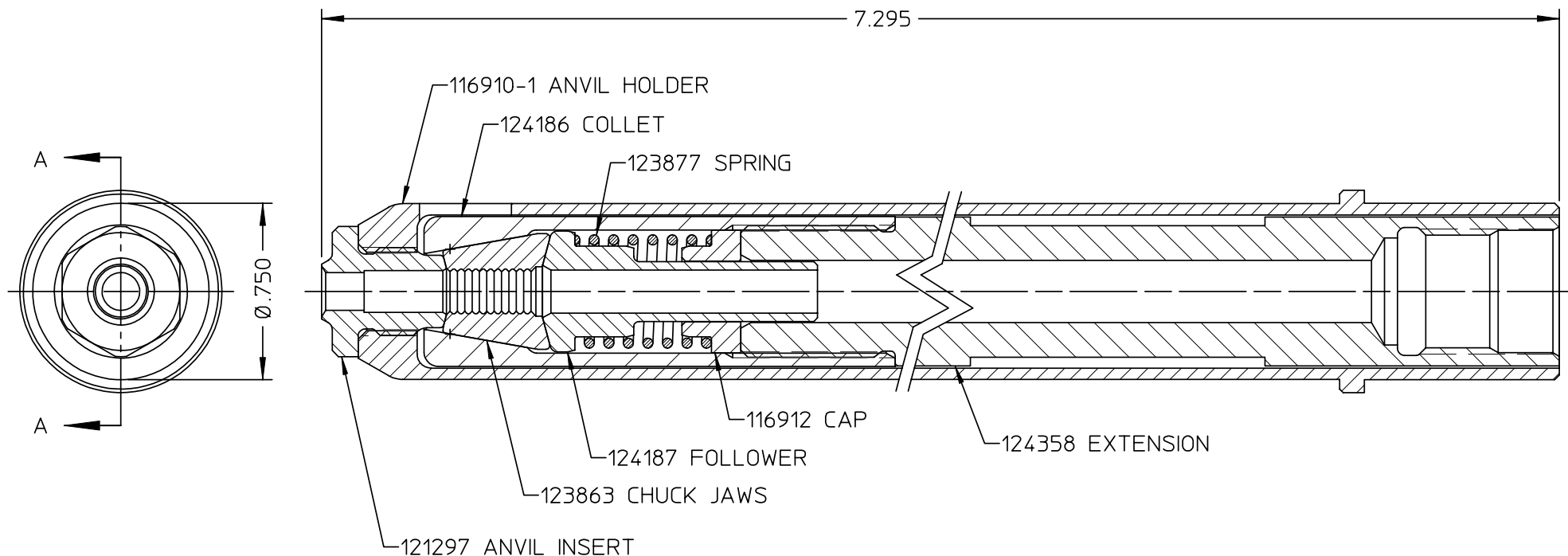
SECTION A-A
