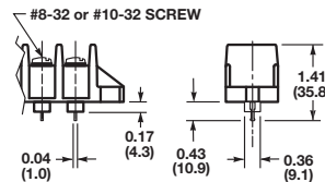
A4013XX (#8-32) A4043XX (#10-32)
