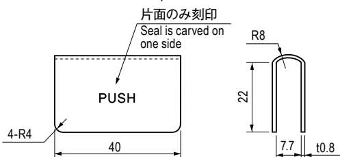
TL-134-3 受金具 Keeper
