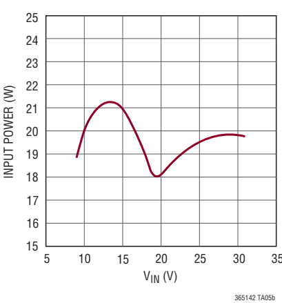
Input Power vs VIN
