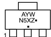
SOT-223 ST SUFFIX CASE 318E
