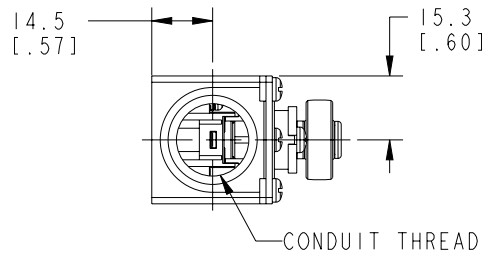
Figure 11. GLC Conduit
