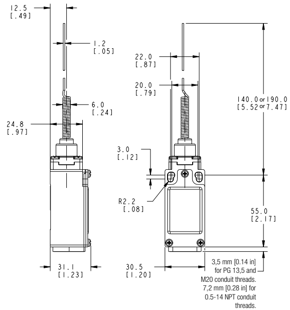
Figure 11. GLC Conduit
