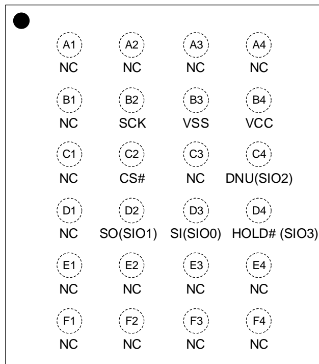
24-ball TFBGA
