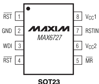
SOT23
