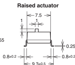
Flat actuator
