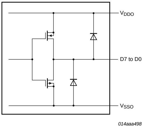
Fig 10. CMOS data outputs
