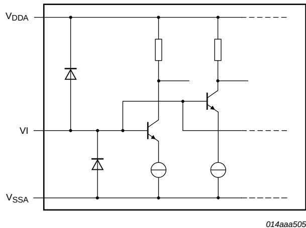
Fig 11. VI analog input
