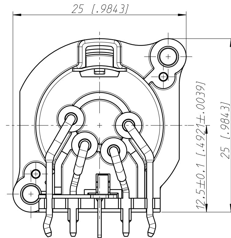
min. Einbauabstand min. assembling distance M 1:1
