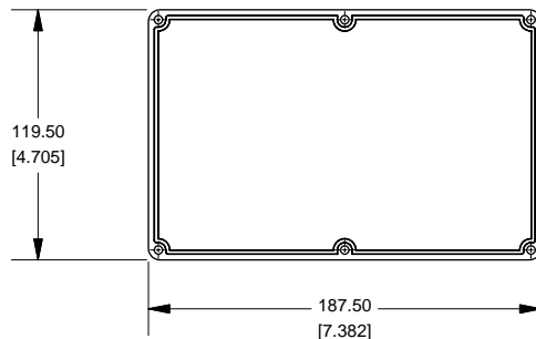
Lid
