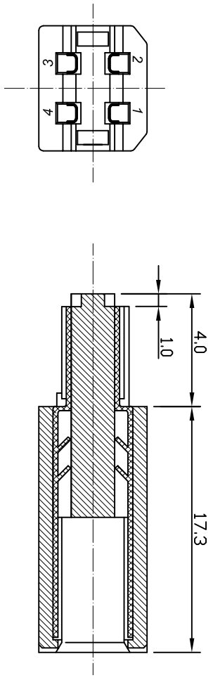
SECTION A-A
