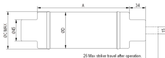
SJ Outline
