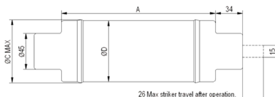
SJ Outline
