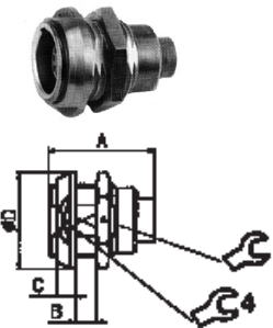
EA : Double nut
