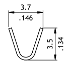
SEC: A-A
