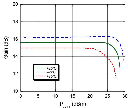
P1dB
