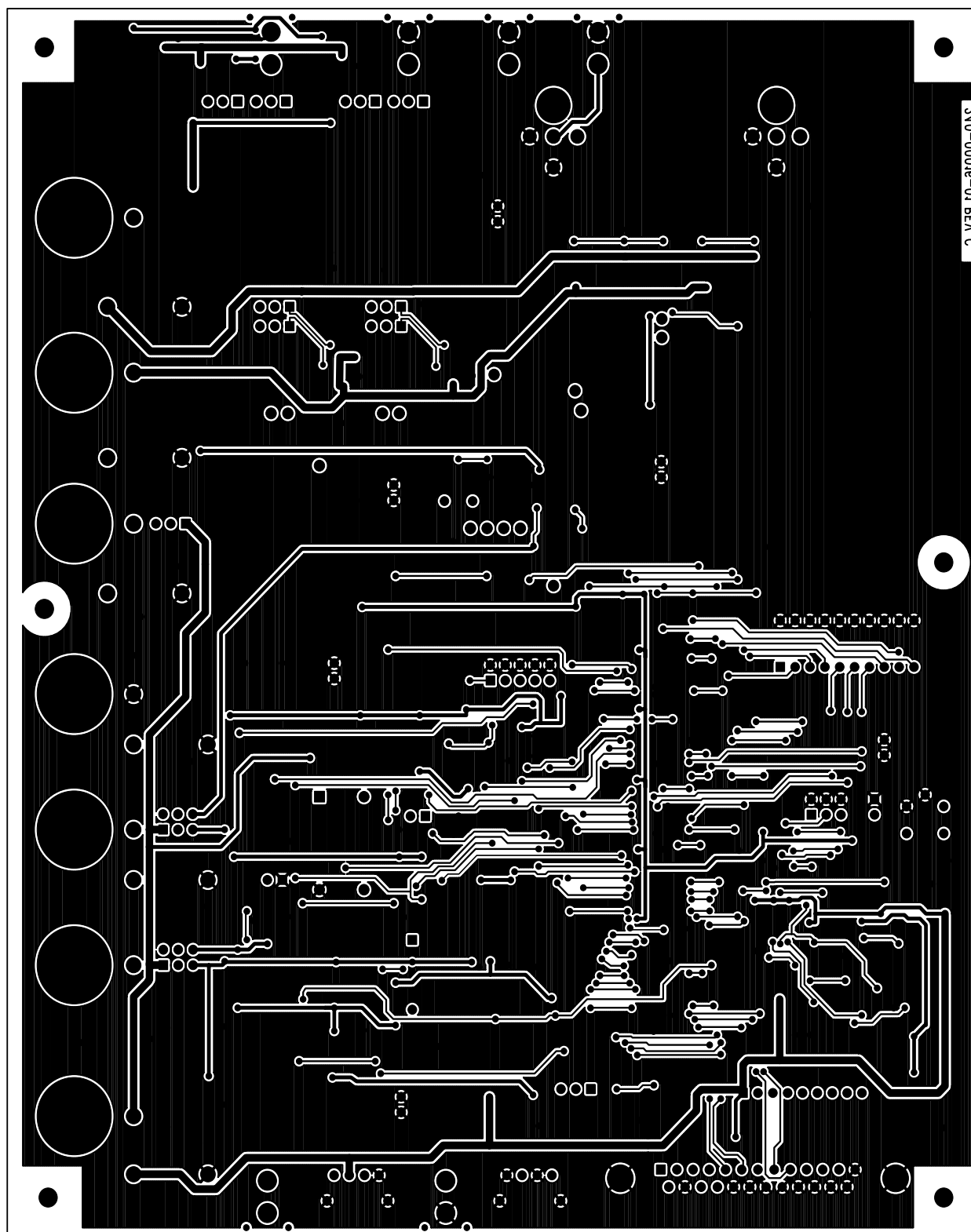
Figure 18. Bottom Layer
