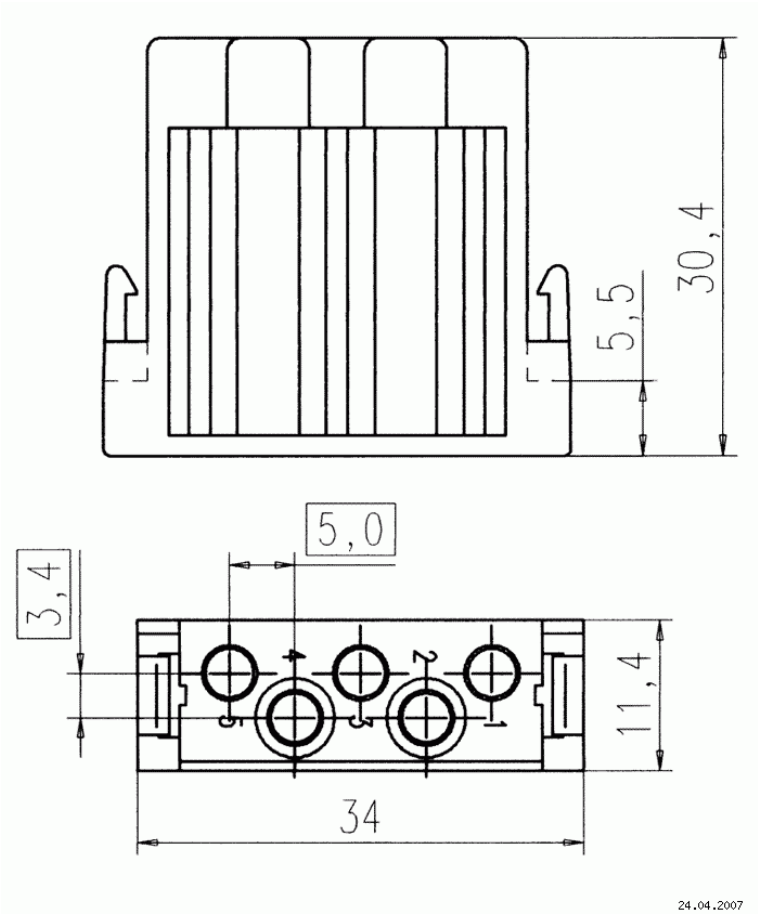
Maßzeichnung Dimensions in mm (Inch)
