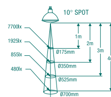
Superia 50 / 35W / 10°
