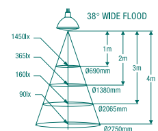
Superia 50 / 35W / 38°
