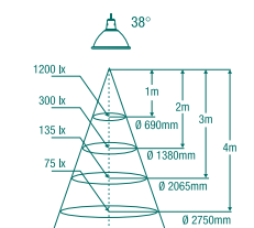
Dichroic 35W / 38°
