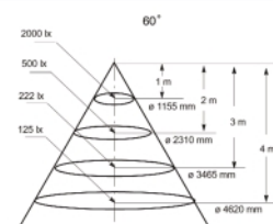
BriteSpot™ ES50 35W 60°
