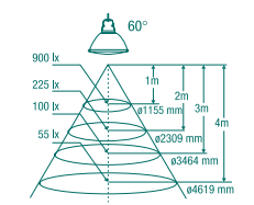
Coolfit 50W / 60°
