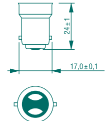
B15d/SBC
