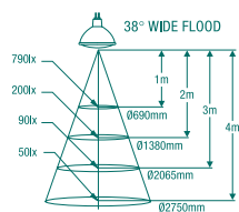
Superia 50 / 20W / 38°
