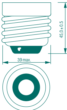
E40/GES
