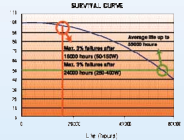
SHP-TS TWINARC
