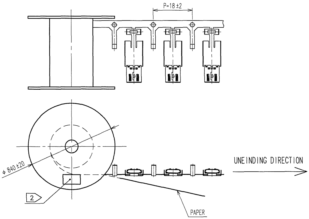
Fig - 1 REELING(FREE)
