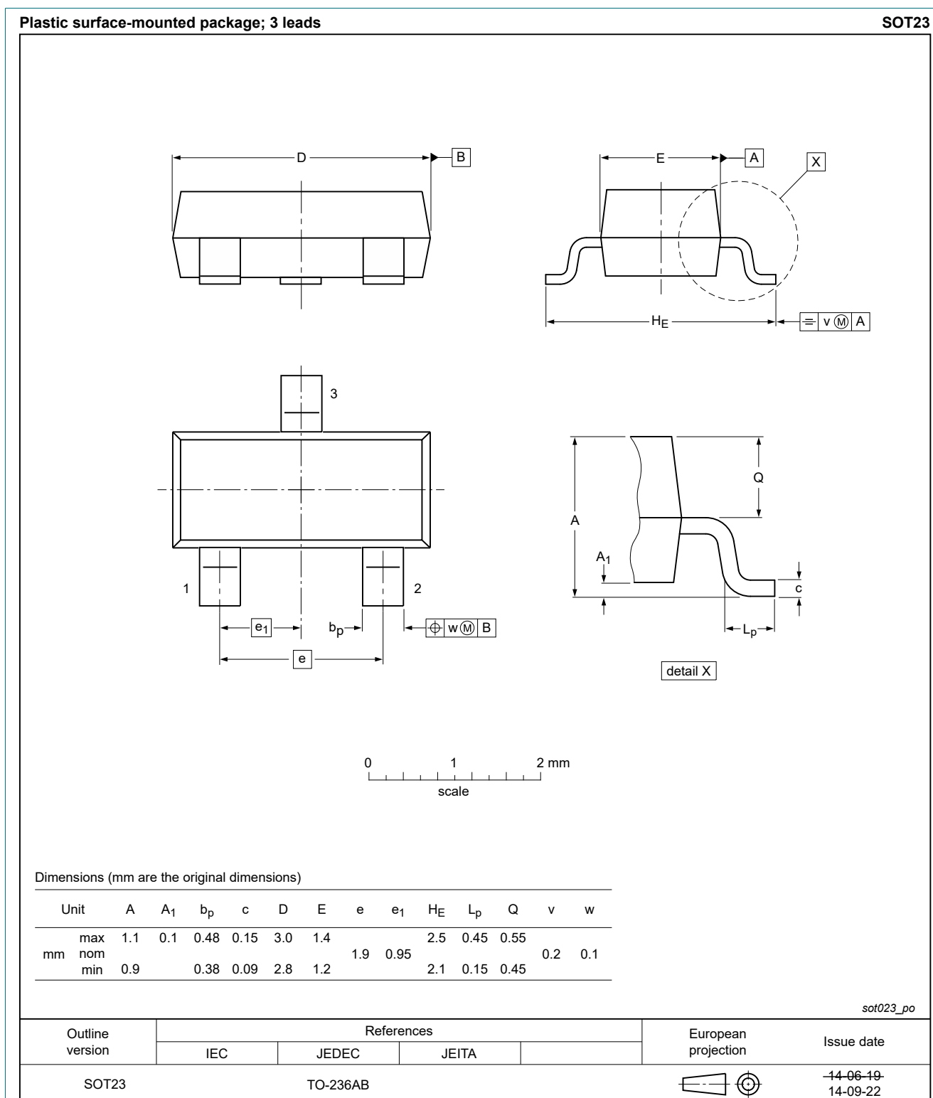
Fig. 14. Package outline SOT23
