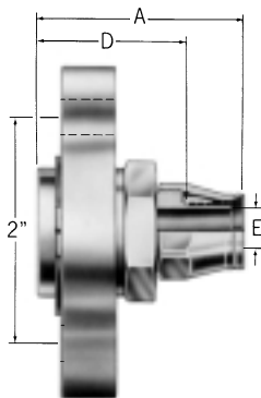
2-bolt swivel flange 63-190626-
