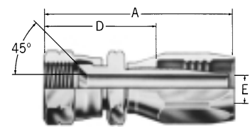
SAE 45° swivel 4401-
