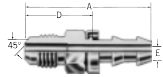
SAE 45° male flare 4742-
