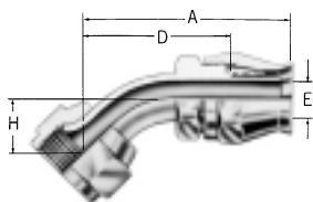
45° elbow 190773- Universal FC9341- SAE 45° swivel
