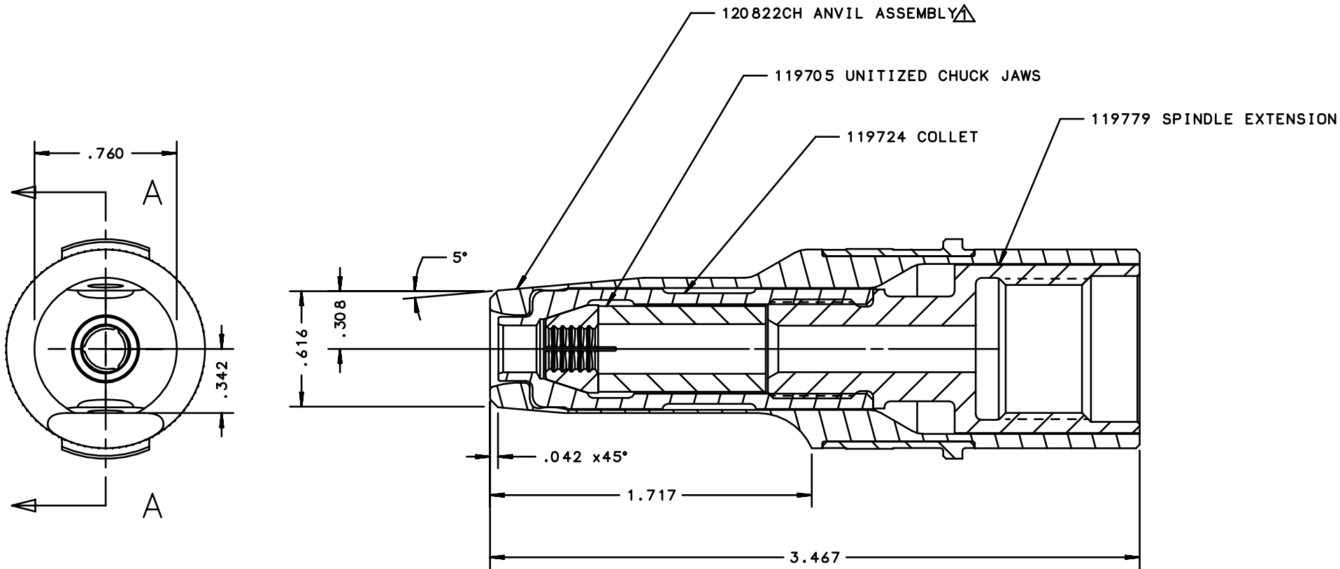
SECTION A-A
