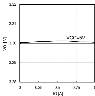
Fig.17 IO-VO (VO=3.3V)
