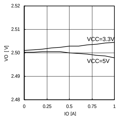
Fig.16 IO-VO (VO=2.5V)
