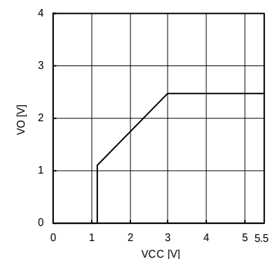
Fig.18 VCC-VO (IO=0A)
