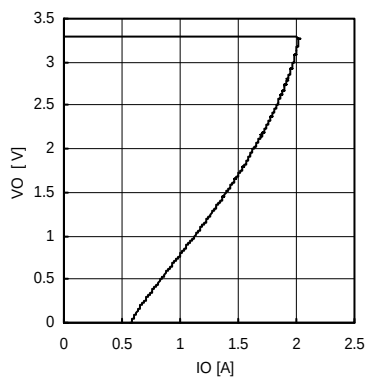
Fig.20 OCP (VCC=5V, VO=3.3V)
