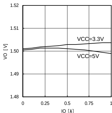
Fig.14 IO-VO (VO=1.5V)
