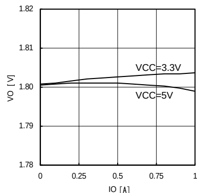
Fig.15 IO-VO (VO=1.8V)
