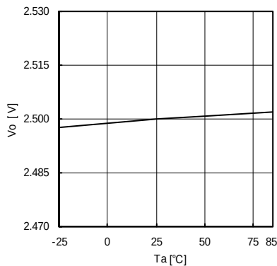
Fig.8 Ta-VO (IO=0A)
