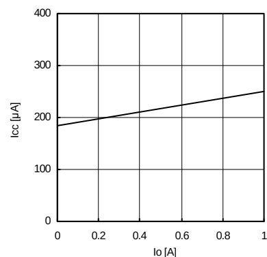
Fig.30 IO-ICC
