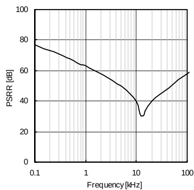
Fig.31 PSRR(IO=0A)
