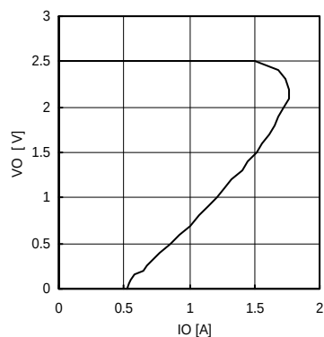
Fig.25 OCP (VCC=3.3V, VO=2.5V)
