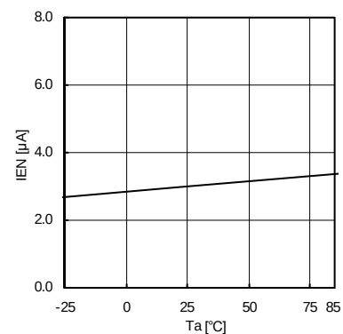
Fig.12 Ta-IEN
