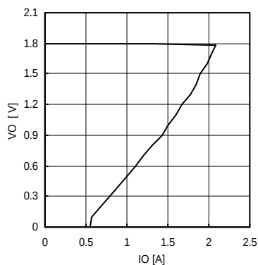
Fig.26 OCP (VCC=3.3V, VO=1.8V)
