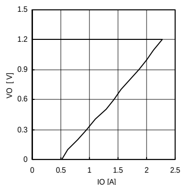
Fig.28 OCP (VCC=3.3V, VO=1.2V)
