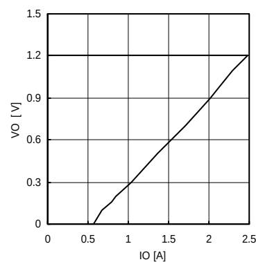
Fig.24 OCP (VCC=5V, VO=1.2V)
