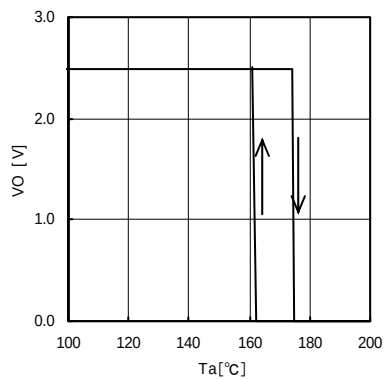
Fig.19 TSD (IO=0A)
