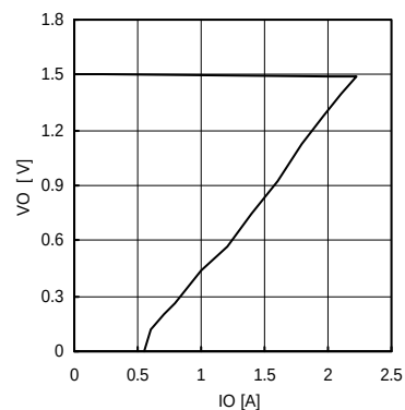
Fig.27 OCP (VCC=3.3V, VO=1.5V)
