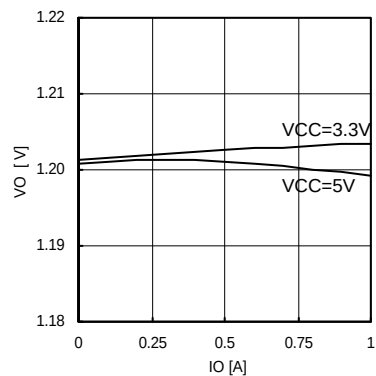
Fig.13 IO-VO (VO=1.2V)
