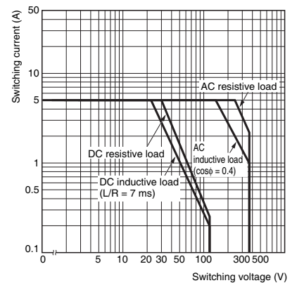
G2R-1Z4, G2R-1AZ4
