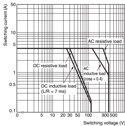
G2R-24, G2R-2A4
