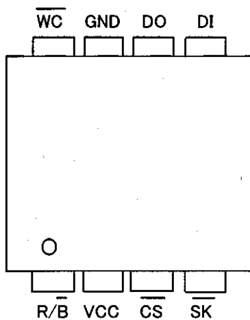
BR9010FV-W:SSOP8 BR9010F-W:SOP8
