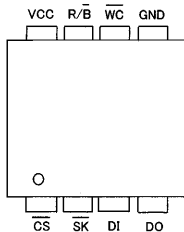
BR9010RFVM-W:MSOP8 BR9010RFV-W:SSOP8
