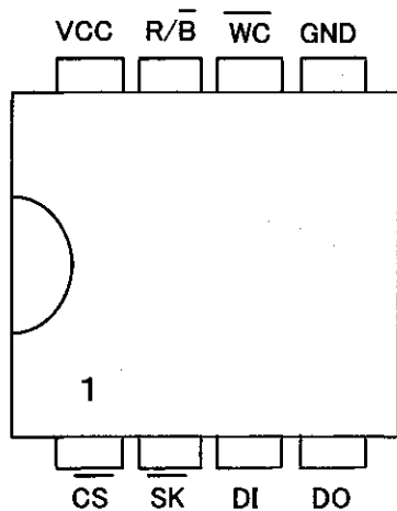
BR9010-W:DIP8
