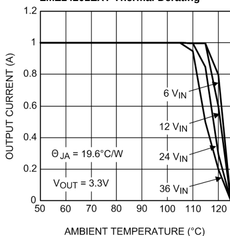
LMZ14201EXT Thermal Derating
