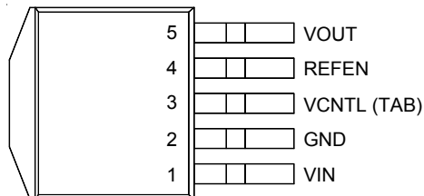
TO-263-5 (RT9173A)
