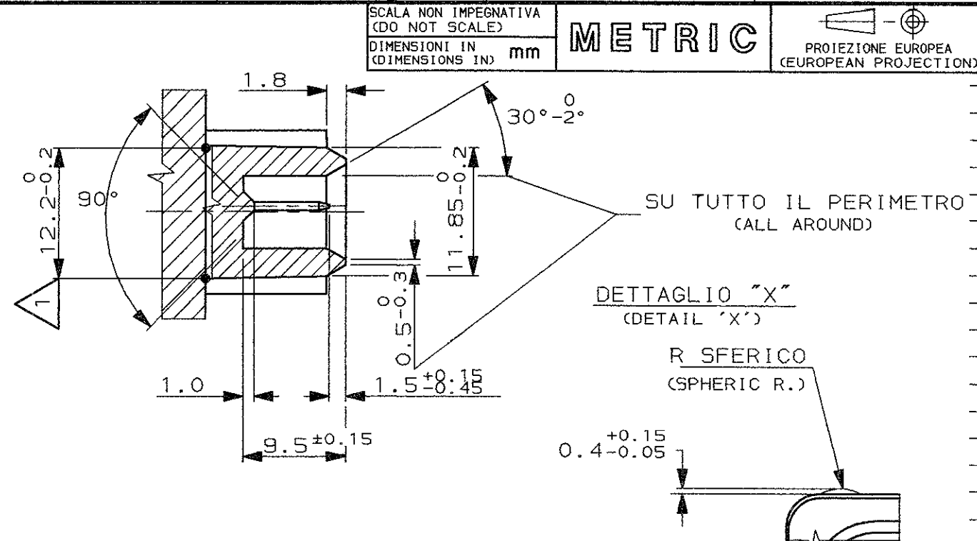
DETT. TAB - SCALA 5:1 (TAB DETAIL)
