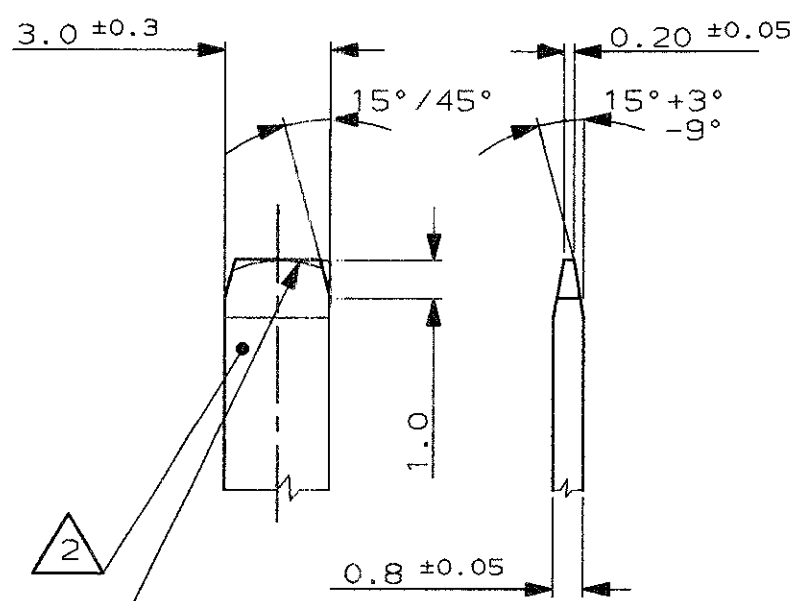
DETT. TAB - SCALA 5:1 (TAB DETAIL)
